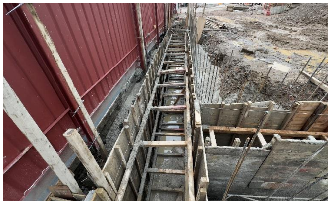
預壘樁施作
