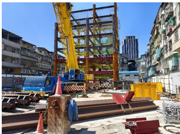
鋼結構安裝
