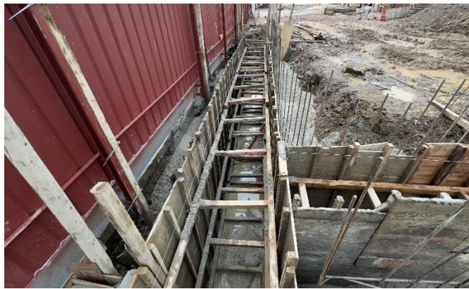
預壘樁施作
